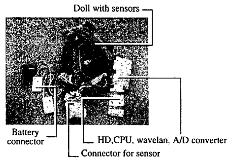
図 4: ぬいぐるみ内部の設置状況
