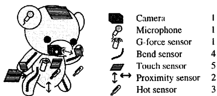
図 5: センサの設置
