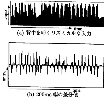
図 9: 背中の圧力センサからの値の例
