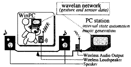
図 3: システム構成
